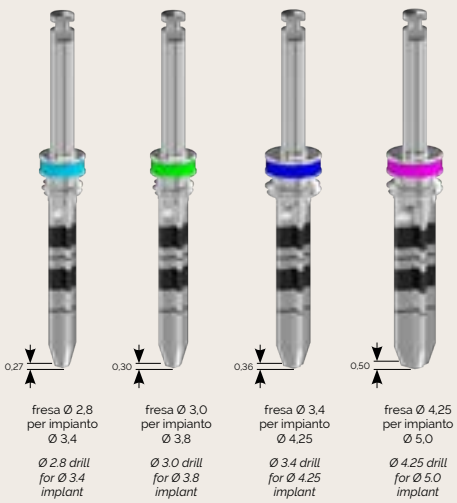
Lunghezza punte frese - Length of drill tips
